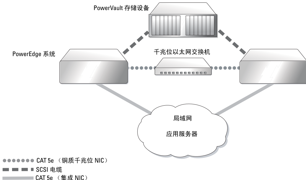
图 2-2. SCSI 群集的硬件连接
